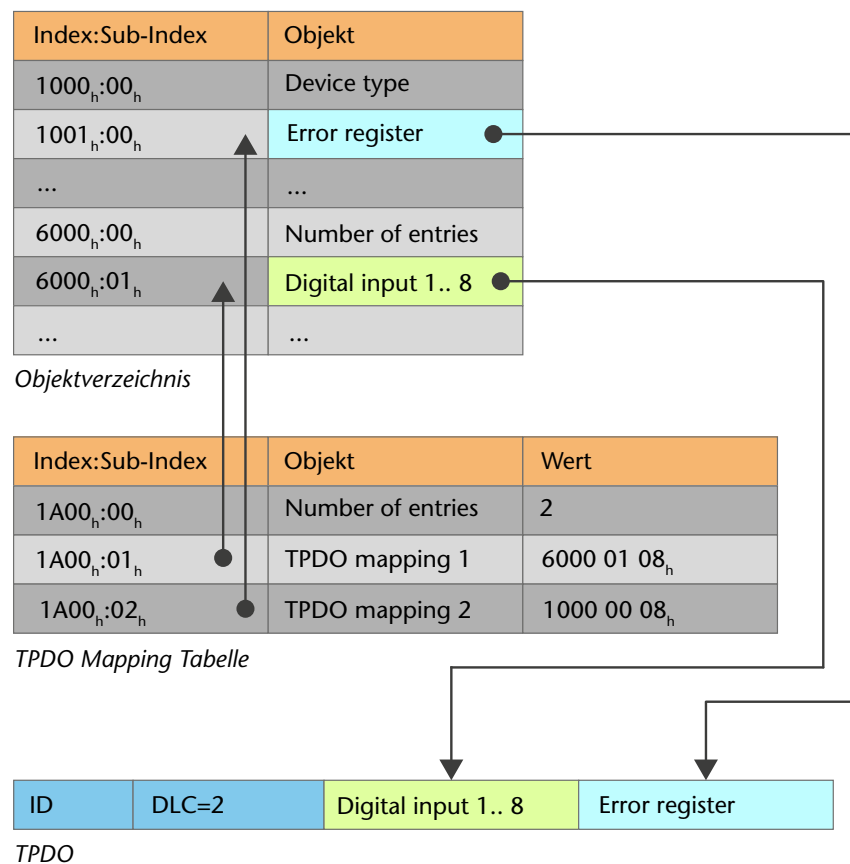
Abb. 5: Verwendung der PDO Mapping Tabelle
