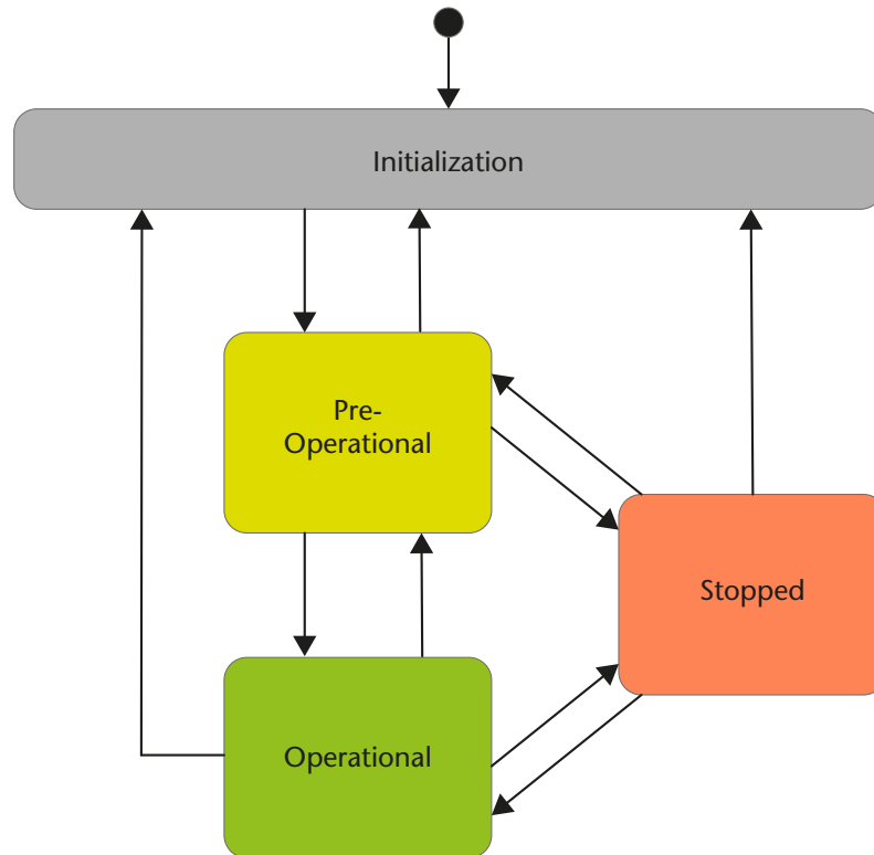
Abb. 6: NMT Zustandsdiagramm
