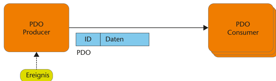
Abb. 3: Ereignis-gesteuerte PDO
